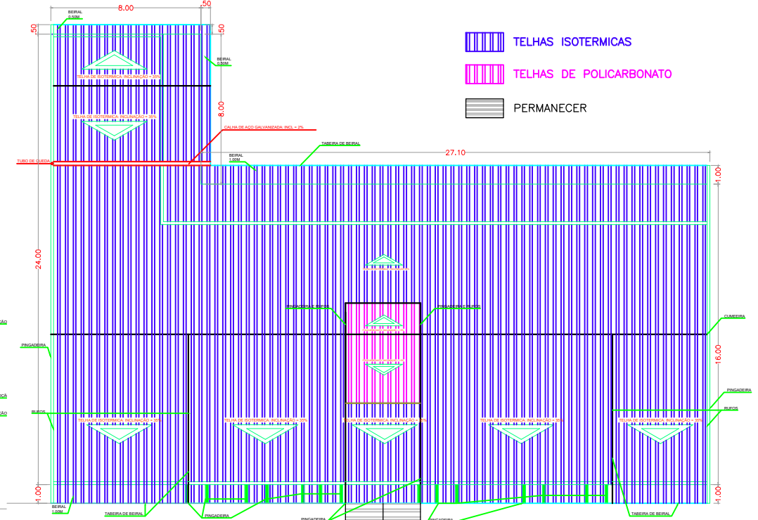
2 PLANTA DE COBERTURA NOVA
