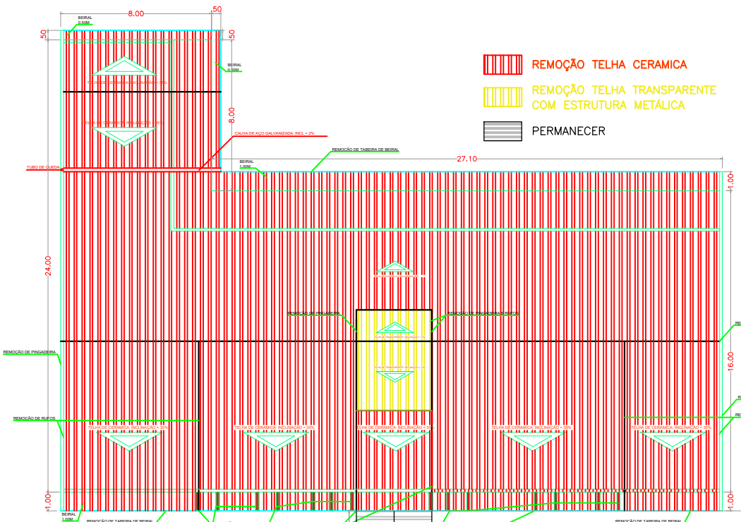
1 PLANTA DE COBERTURA EXISTENTE - REMOÇÃO
